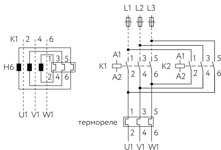
Главная цепь:
