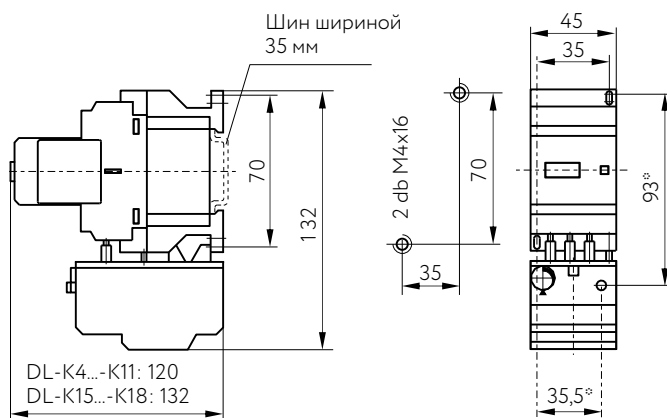
DL-K4...DL-K18+H0-2K моторстартер
