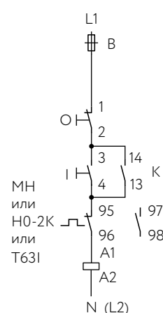
Управляющая цепь
