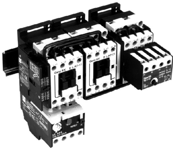
Csillag-háromszög motorvédő kombináció
