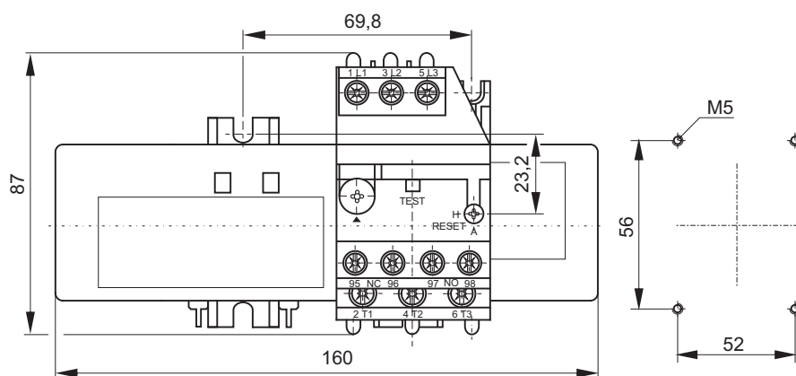
H6 típusú áramváltós hőrelé
