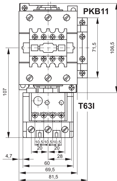
DL-K22...DL-K37 + T63I dugaszolt motorvédő kombináció
