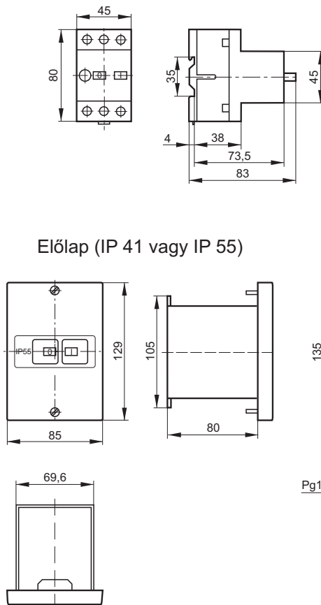
GMV 25f nyomógombos motorvédő kapcsoló
