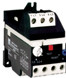
H0-2K hőrelé, adapteres kivitel
