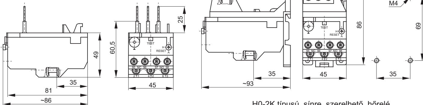
H0-2K típusú, sínre szerelhető hőrelé
