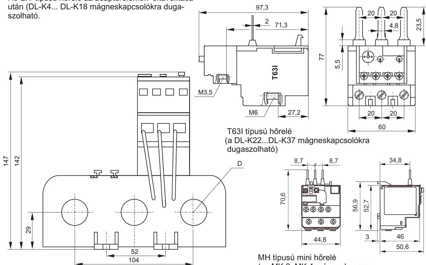
H0-2K típusú, sínre szerelhető hőrelé
