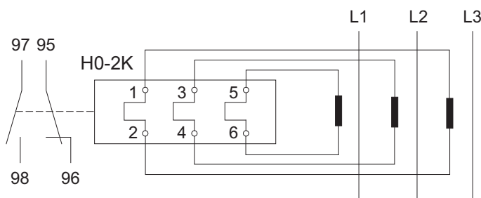
A kapcsolás vázlatja
