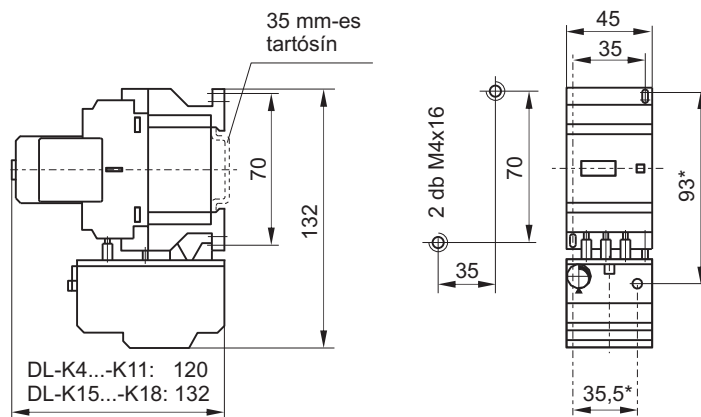
DL-K4...DL-K18+H0-2K dugaszolt kombináció
