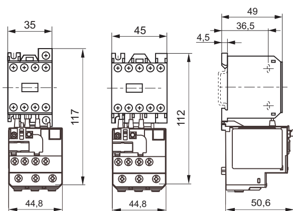
MK + MH dugaszolt motorvédő kombináció
