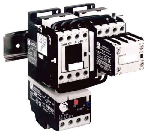
Irányváltó motorvédő kombináció
