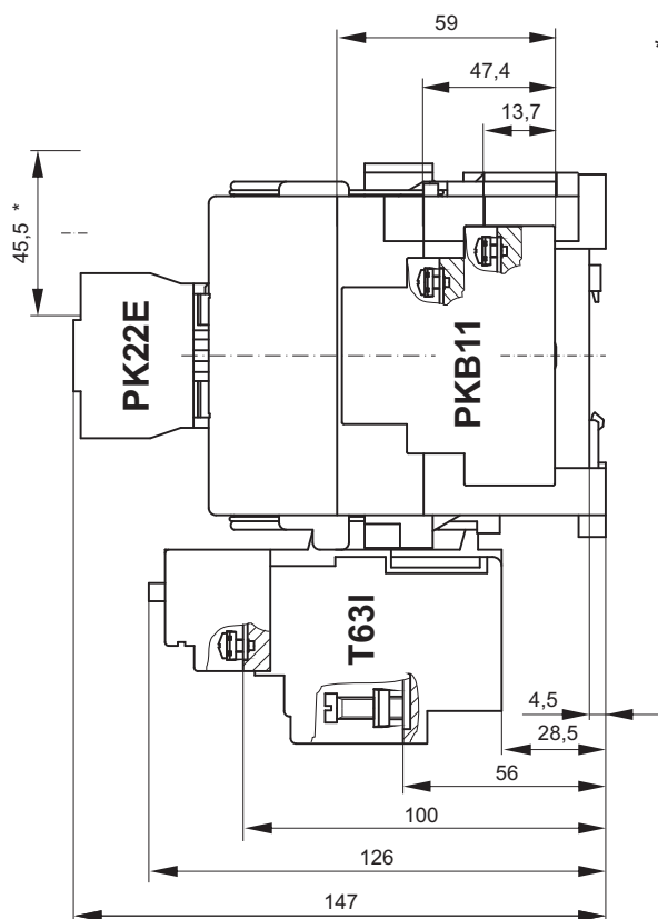
DL-K22...DL-K37 + T63I dugaszolt motorvédő kombináció
